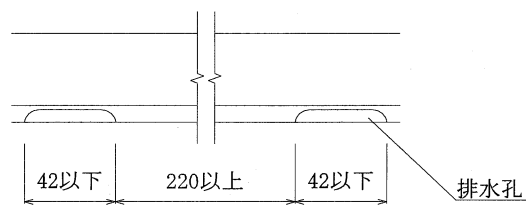
背面図
