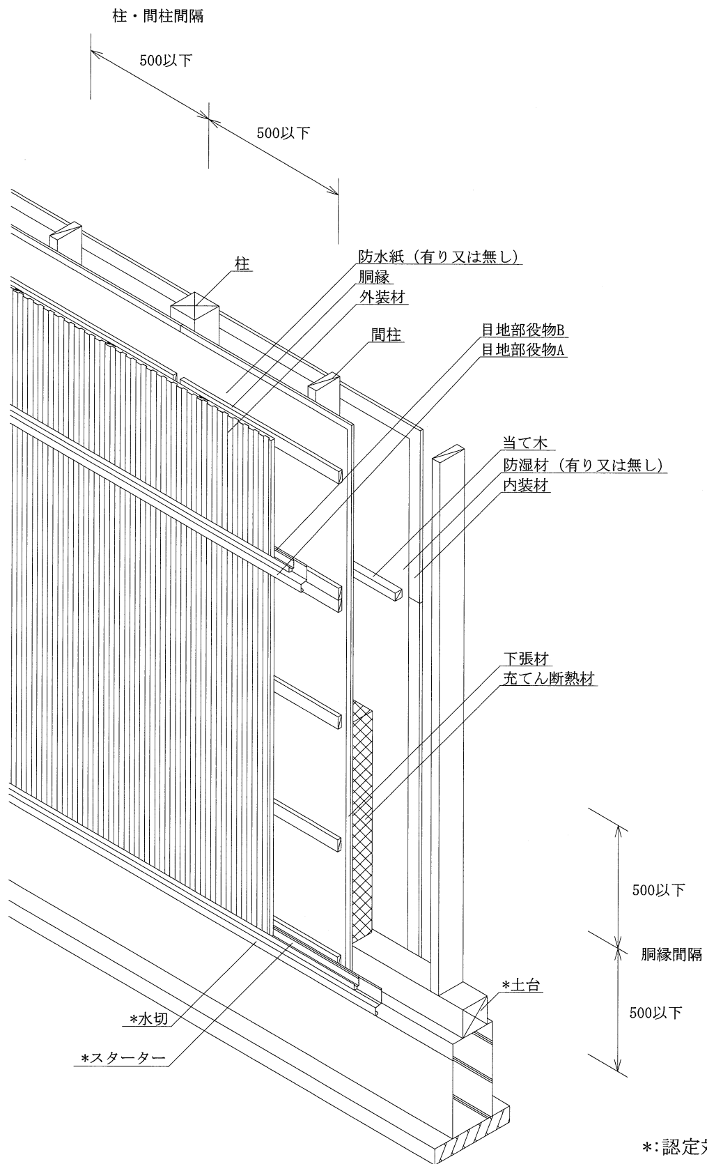
透視図
