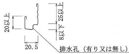
断面詳細図
