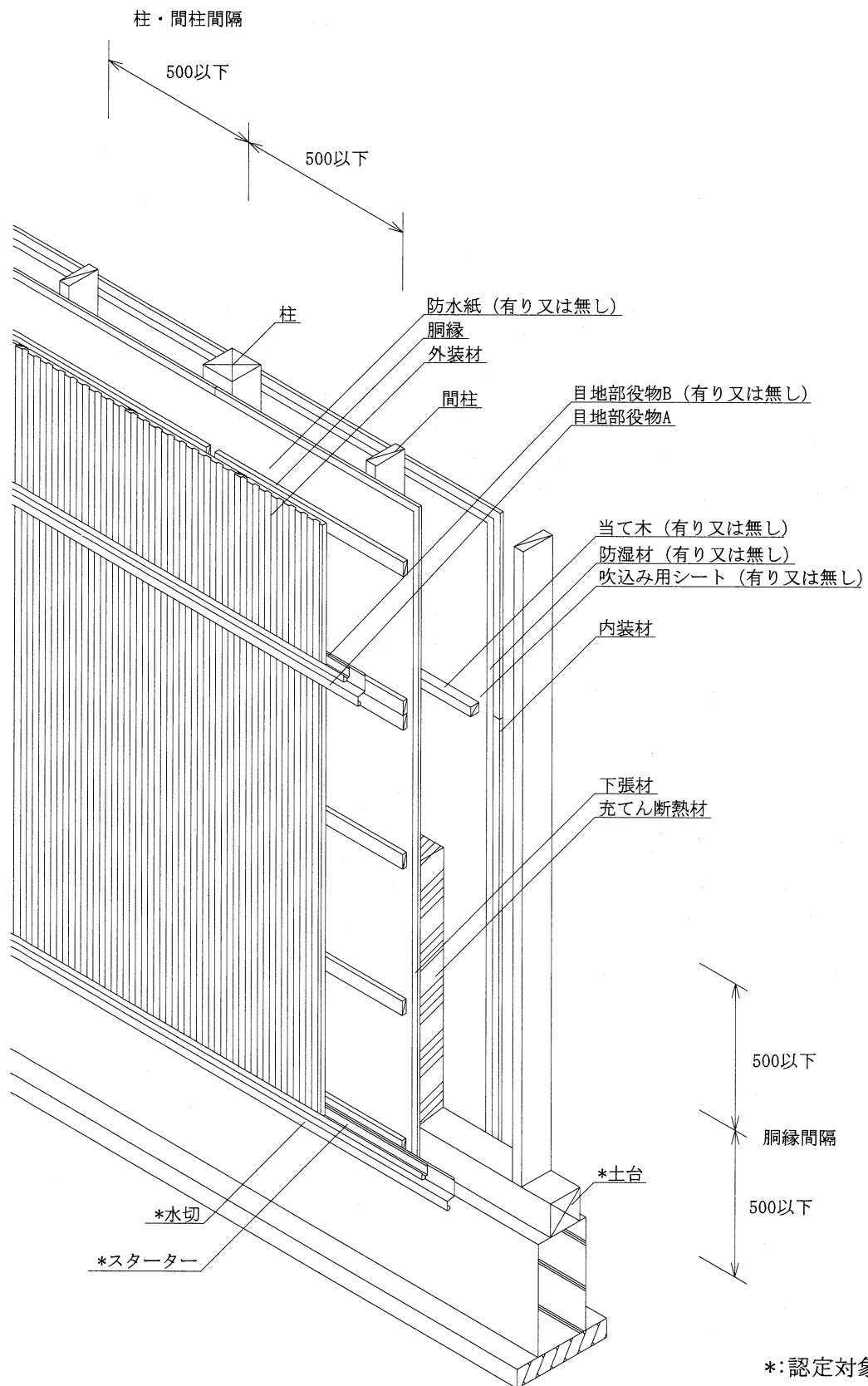
透視図 (別添 - 15)
