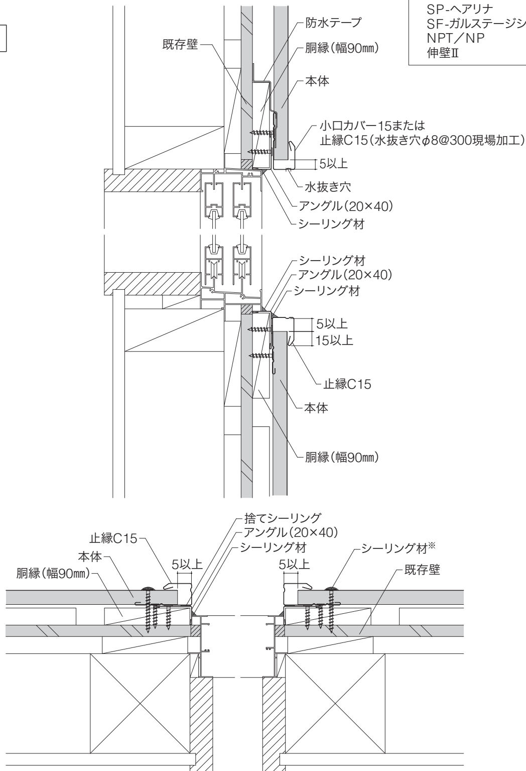
断面図
