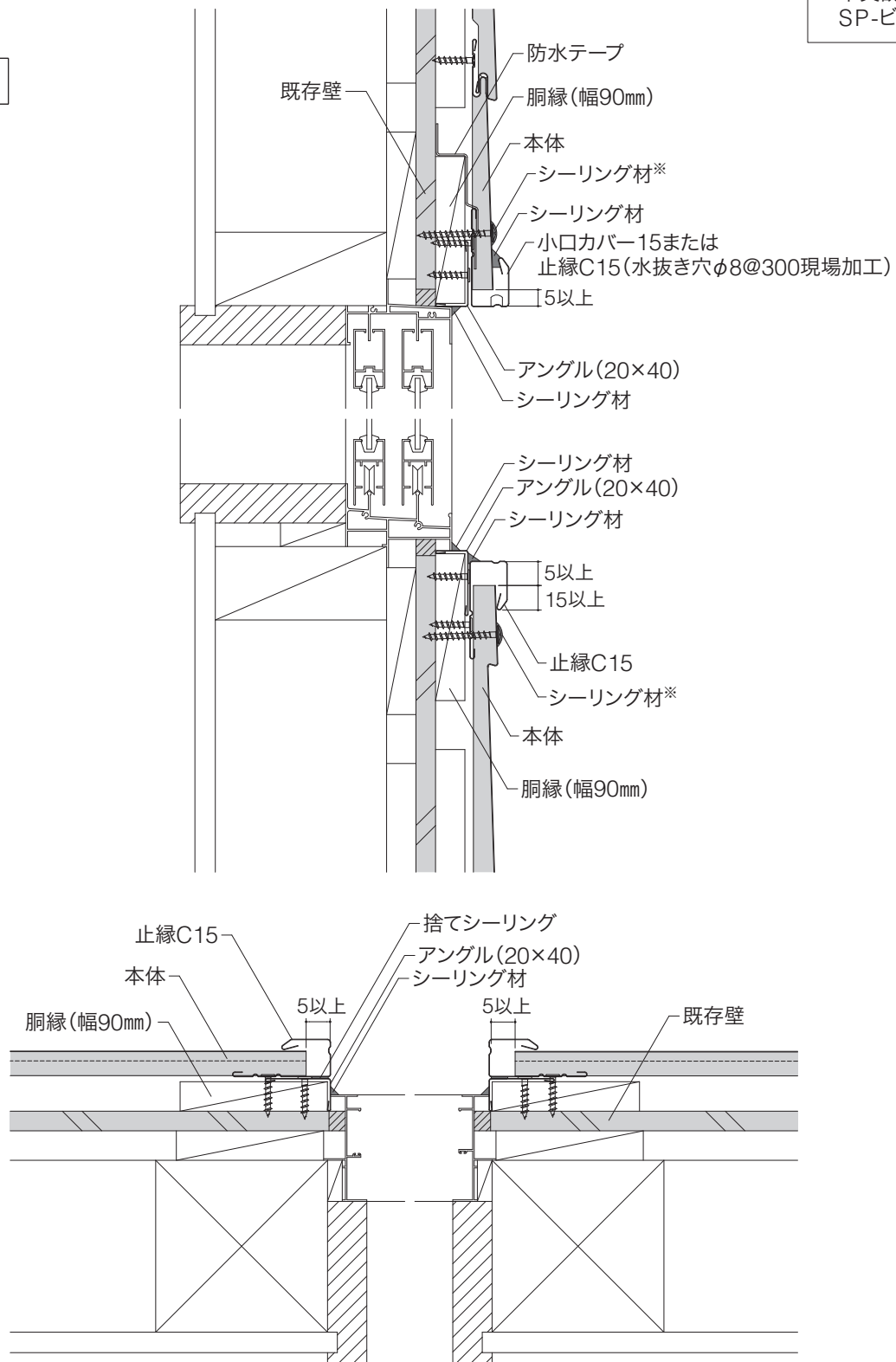
断面図
